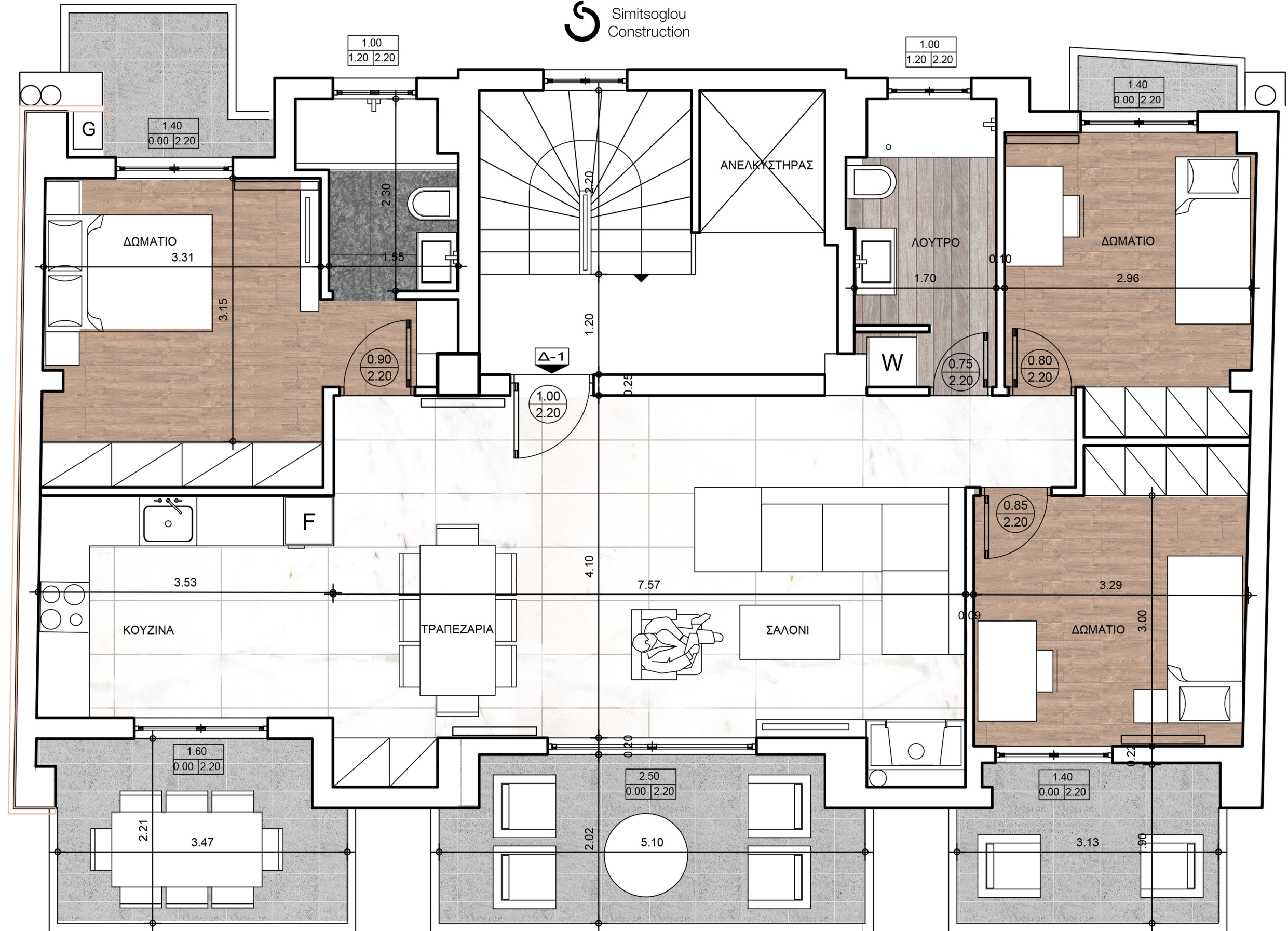
Κάτοψη 4ου ορόφου
